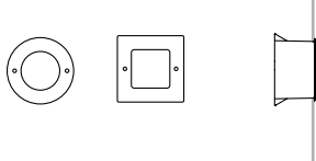
T1/T1: Ø 148(L,W) x 93(H) mm Q1/Q1: 148x148 (L,W) x 93(H) mm
