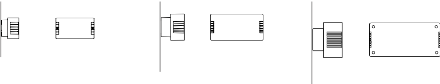
MICRODUPLO/Q 192(L) x 98(W) x 104(H) mm MINIDUPLO/Q 275(L) x 139(W) x 140(H) mm DUPLO/Q 367(L) x 171(W) x 176(H) mm
